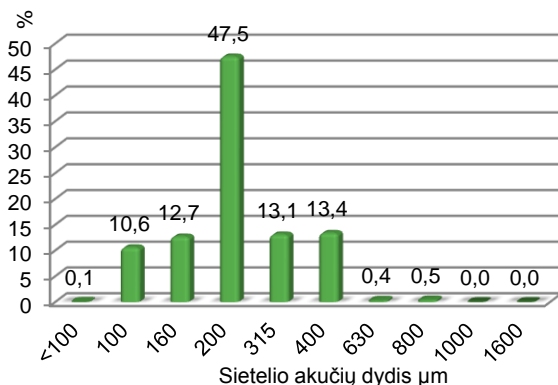
GRANULIOMETRINĖ ANALIZĖ
