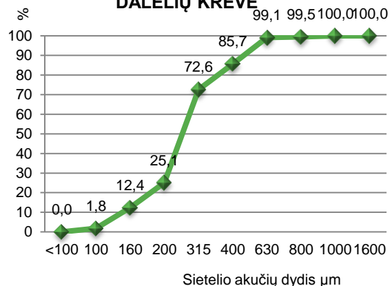
DALELIŲ KREIVĖ
